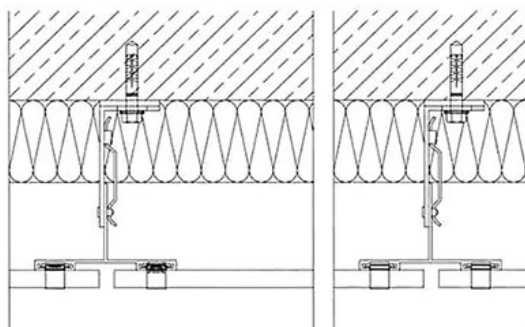
Sistema di facciata ventilata con montanti verticali
