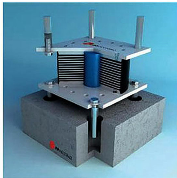
ISOLATORE IN GOMMA E PIOMBO
